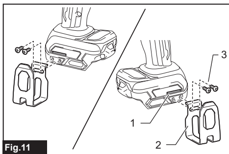
► 1. Groove 2. Hook 3. Screws
